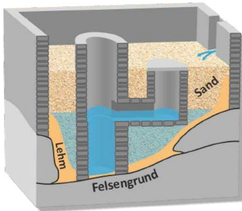
Zeichnung der Zisternenkammer
